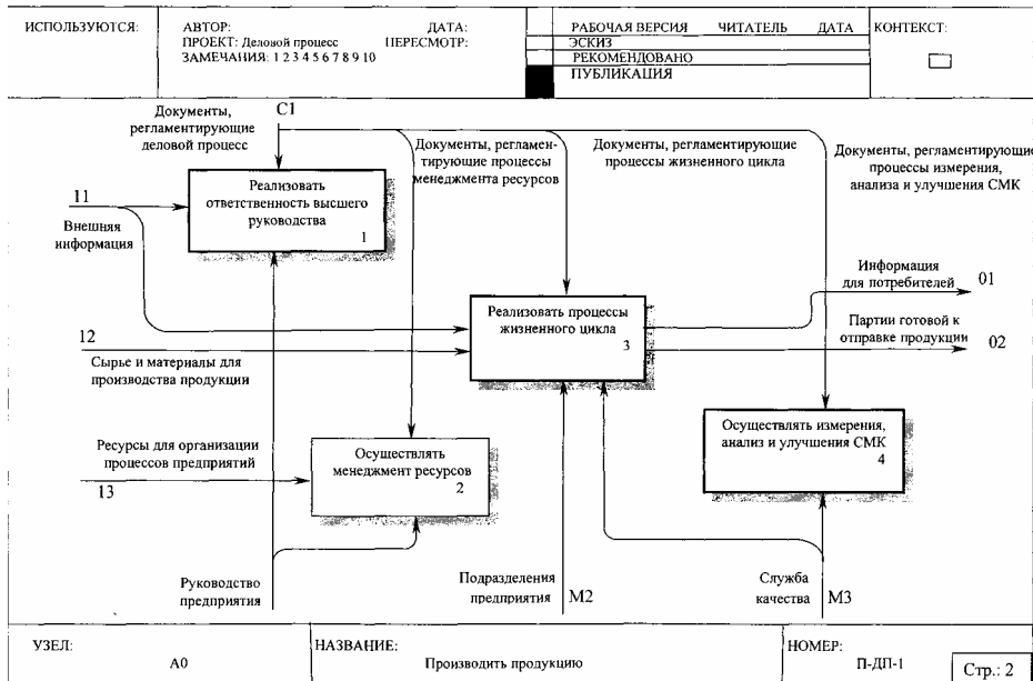
Вернуться в каталог учебников Рис. 22. Деконпозиция процесса «Производить продукцию» http://учебники.информ2000.рф/учебники.shtml Обозначение: П1, П2, П3 – входы, О1, О2 – выходы, С1 – управление, М1, М2, М3 – механизмы
