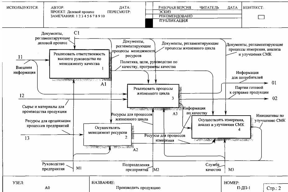
Возвращение в каталог учебников Рис. 24. Декомпозиция процесса «Производство продукции» для взаимодействия между процессами http://учебники.информ2000.рф/учебники.shtml
